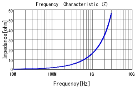
■ LQG15HS2N7C02 |Z|
