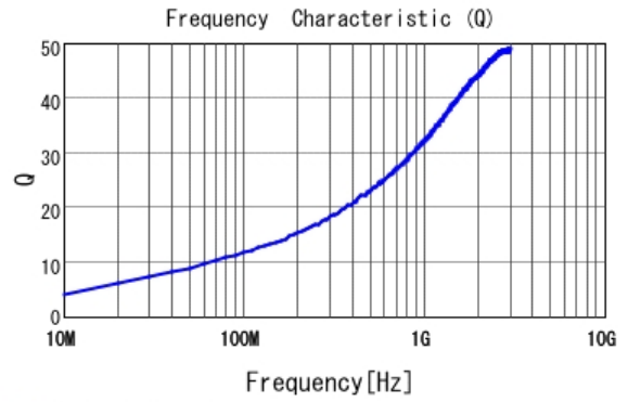
■ LQG15HS2N7C02 Q
