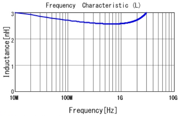
■ LQG15HS2N7C02 L
