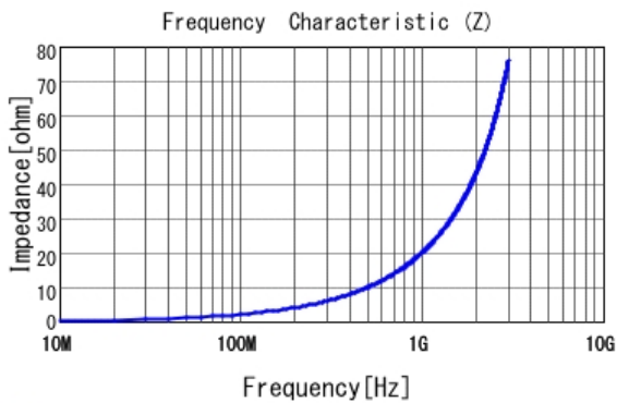
■ LQG15HZ3N3C02 |Z|
