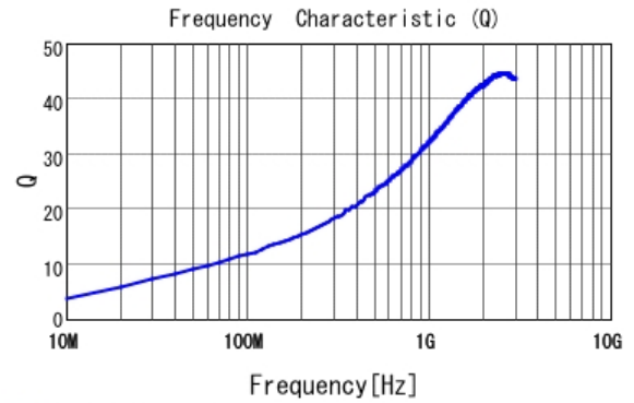
■ LQG15HZ3N3C02 Q
