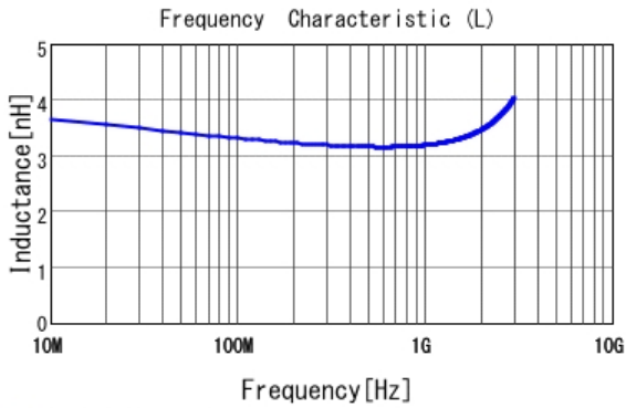
■ LQG15HZ3N3C02 L
