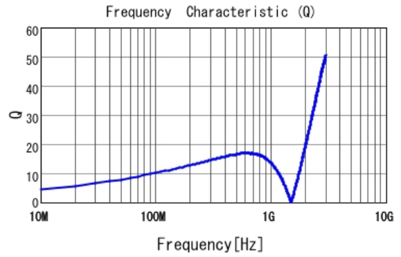
■ LQG15HZ47NJ02 Q
