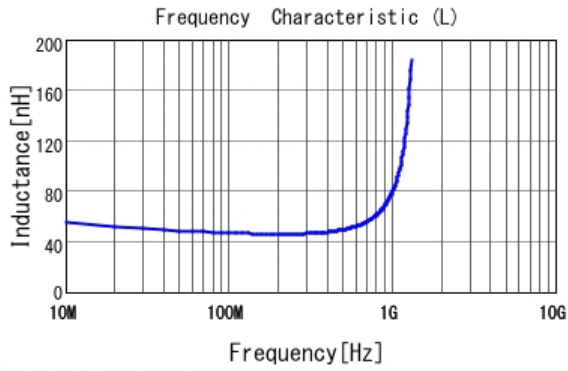
■ LQG15HZ47NJ02 L
