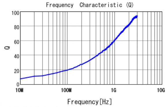
■ LQG15WZ3N3S02 Q
