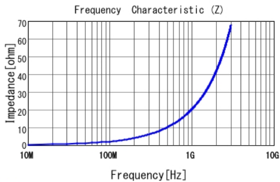
■ LQG15WZ3N3S02 |Z|
