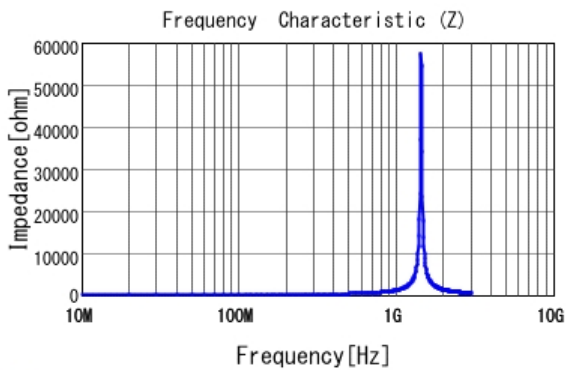
■ LQW2BANR10G00 |Z|
