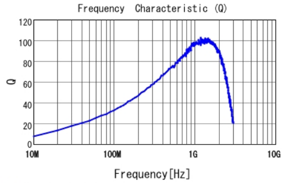
■ LQW2BAS27NJ00 Q
