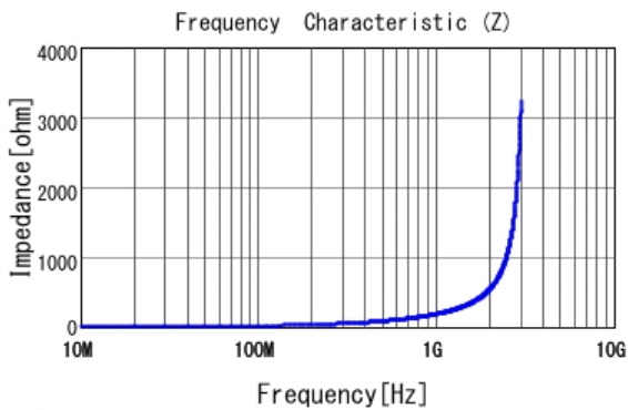
■ LQW2BAS27NJ00 |Z|
