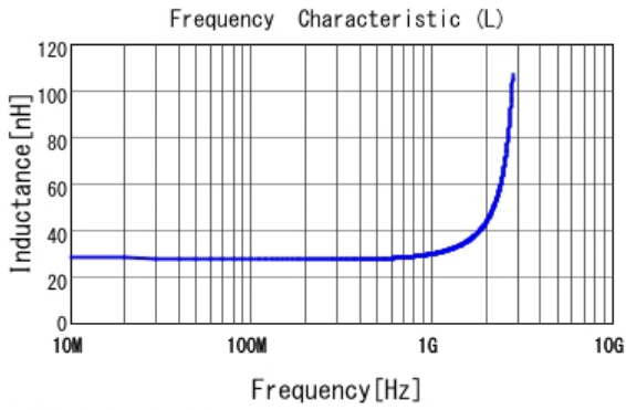
■ LQW2BAS27NJ00 L
