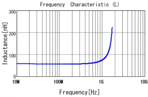
■ LQW2BAS56NG00 L
