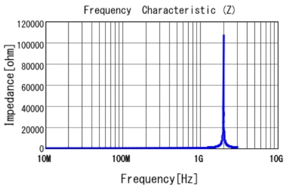
■ LQW2BAS56NG00 |Z|
