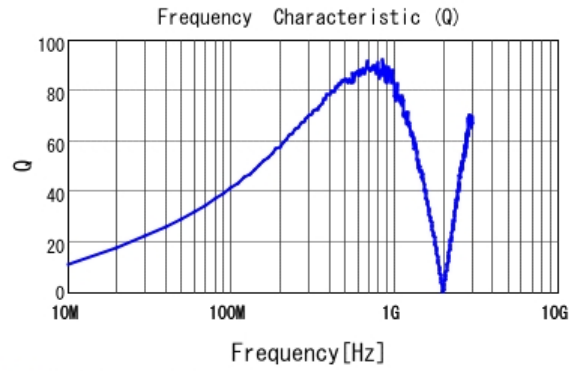
■ LQW2BAS56NG00 Q
