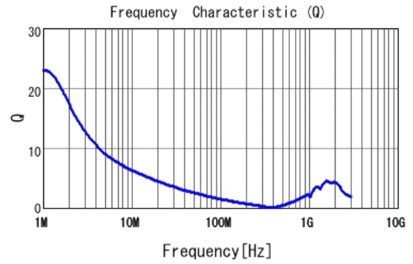
■ LQW32FT2R7M0H Q
