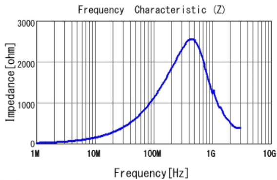
■ LQW32FT2R7M0H |Z|
