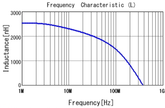
■ LQW32FT2R7M0H L
