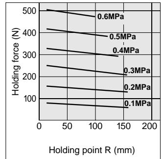
MHL2-40D
