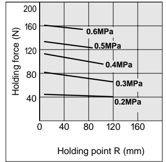
MHL2-40D
