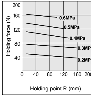
MHL2-40D
