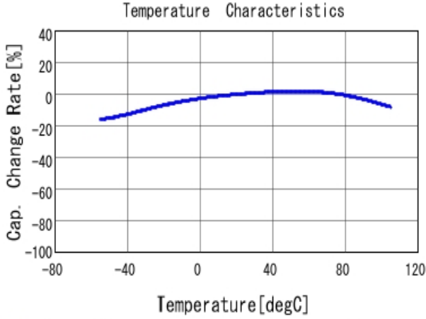
■ GRM033C81A104KE14 C-Temp. capchange, DCO. 0V, ACO. 2V rm
