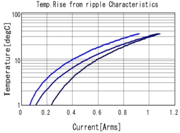
GRM033C81A104KE14 Temp. rise ■ 400kHz ■ 800kHz ■ 1MHz
