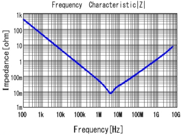
■ GRM155B30J475ME87 |Z| DCOV, 20degC
