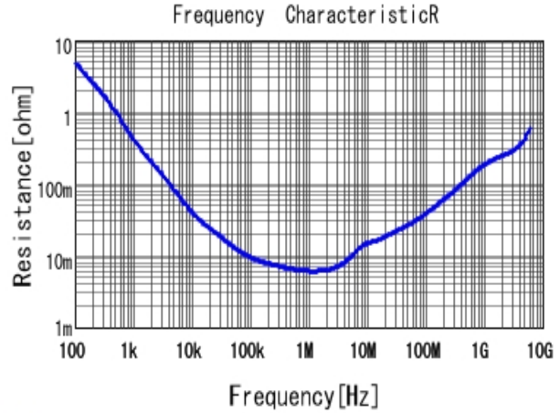
■ GRM155B30J475ME87 R DCOV, 20degC
