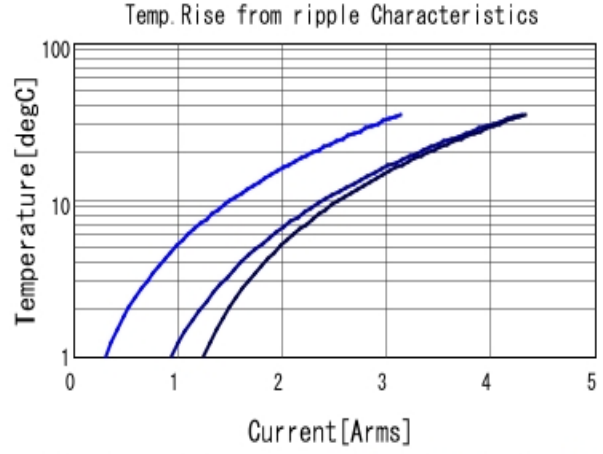
GRM155B30J475ME87 Temp. rise ■ 100kHz ■ 500kHz ■ 1MHz
