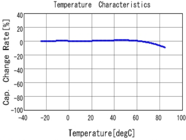
■ GRM155B30J475ME87 C-Temp. capchange, DCO. 0V, ACO. 2V rm
