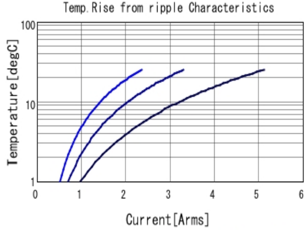
KRM31KR71H475KH01 Temp. rise ■ 50kHz ■ 100kHz ■ 300kHz
