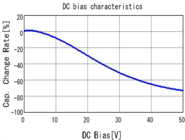
■ GCJ32EC71H106KA01 C-DC bias capchange, 25.0degC, AC1.
