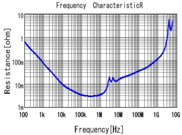
■ GCJ32EC71H106KA01 R DCOV, 25degC
