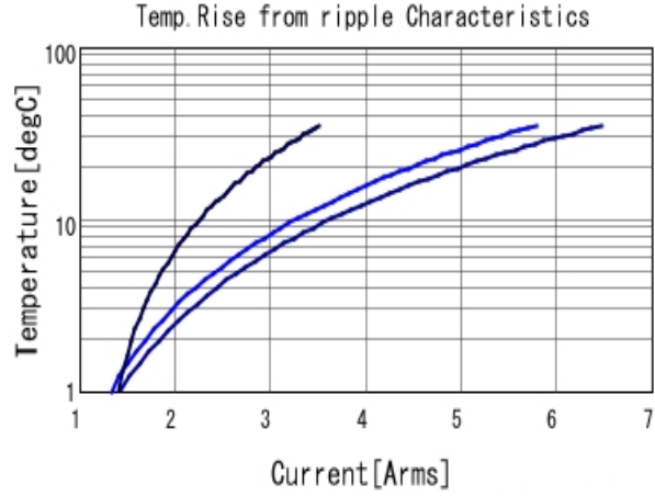
GCJ32EC71H106KA01 Temp. rise ■ 80kHz ■ 400kHz ■ 800kHz
