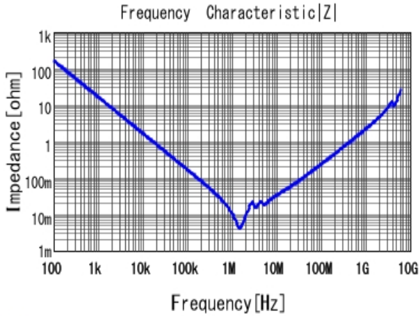
■ GCJ32EC71H106KA01 |Z| DCOV, 25degC
