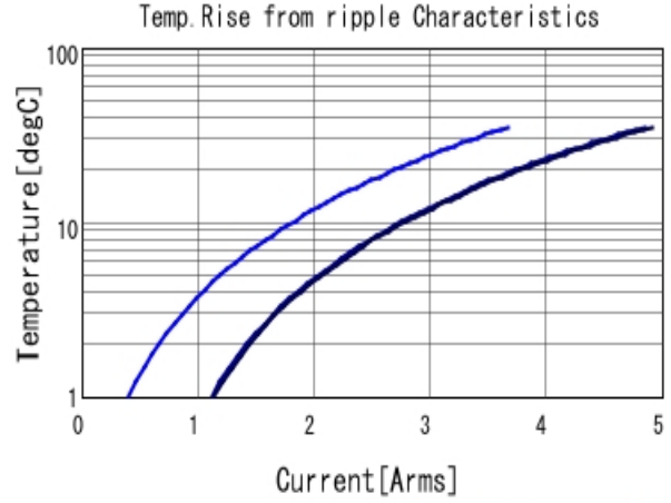
GRM155B30J475ME47 Temp. rise ■ 100kHz ■ 500kHz ■ 1MHz
