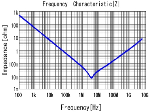
■ GRM155B30J475ME47 |Z| DCOV, 20degC
