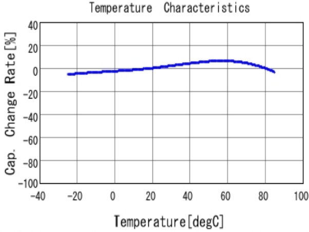
■ GRM155B30J475ME47 C-Temp. capchange, DCO. 0V, ACO. 1V rm
