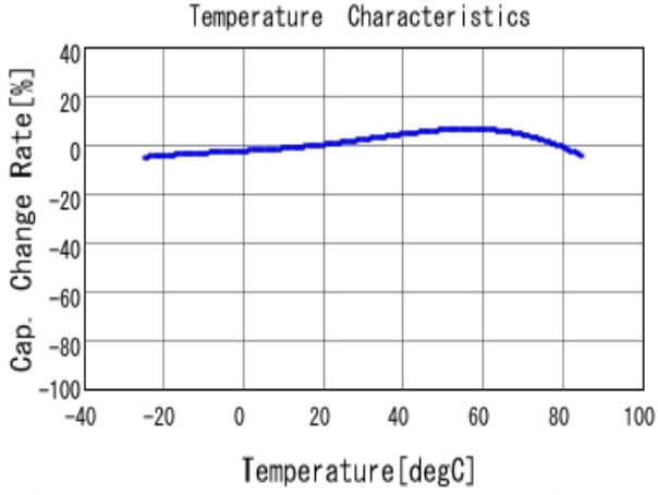
■ GRM155B31A225KE95 C-Temp. capchange, DCO. 0V, ACO. 2V rm
