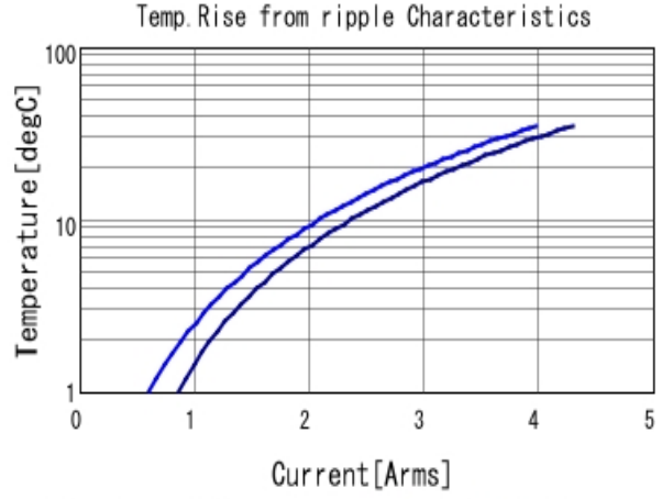
GRM155B31A225KE95 Temp. rise ■ 500kHz ■ 1MHz
