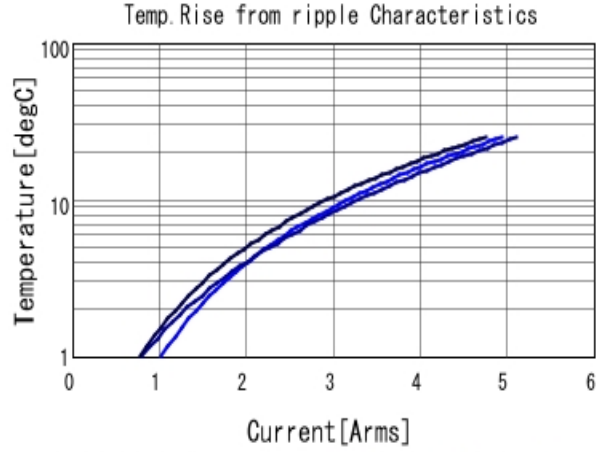
KRM55TR71H226MH01 Temp. rise ■ 50kHz ■ 100kHz ■ 300kHz
