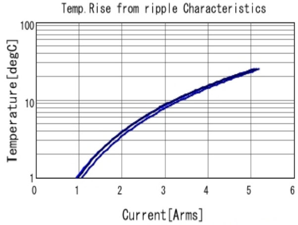
KRM55WR71H336MH01 Temp. rise ■ 50kHz ■ 100kHz ■ 300kHz
