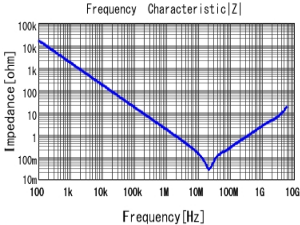
■ GCJ188R71C104KA01 |Z| DC0V, 25degC
