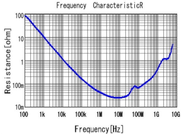
■ GCJ188R71C104KA01 R DC0V, 25degC
