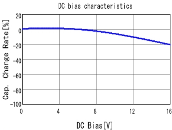
■ GCJ188R71C104KA01 C-DC bias capchange, 25.0degC, AC1.
