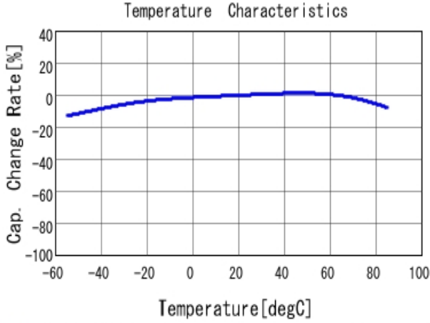
■ GRM033R61A105ME15 C-Temp. capchange, DCO. 0V, ACO. 1Vrm
