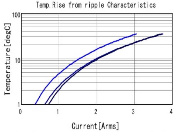
GRT155C80J475ME13 Temp. rise ■ 100kHz ■ 500kHz ■ 1MHz
