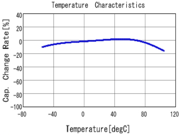
■ GRT155C80J475ME13 C-Temp. capchange, DCO. 0V, ACO. 1V rm
