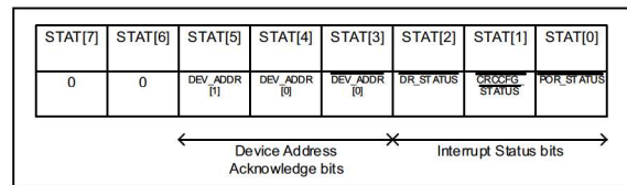
FIGURE 6-1: STATUS Byte.
