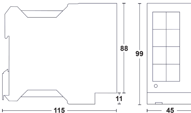
Dimensions : Millimetres
