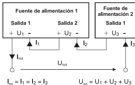
Esquema 2: Modo de funcionamiento en serie
