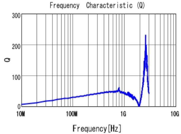
■ LQW15AWR16H80 Q
