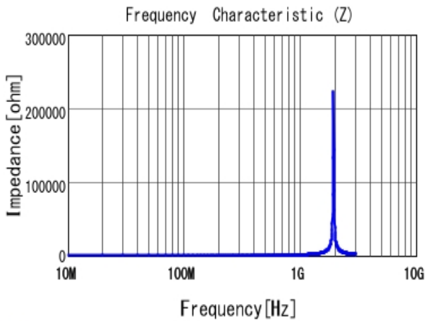
■ LQW15AWR16H80 |Z|
