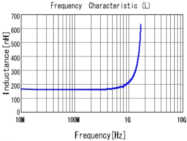
■ LQW15AWR16H80 L
