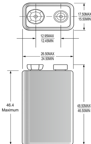
Dimensions : Millimetres
