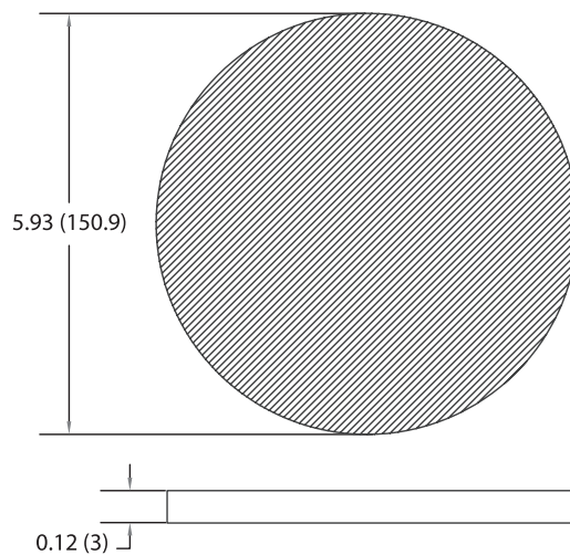
Dimensions : Inches (Millimetres)
