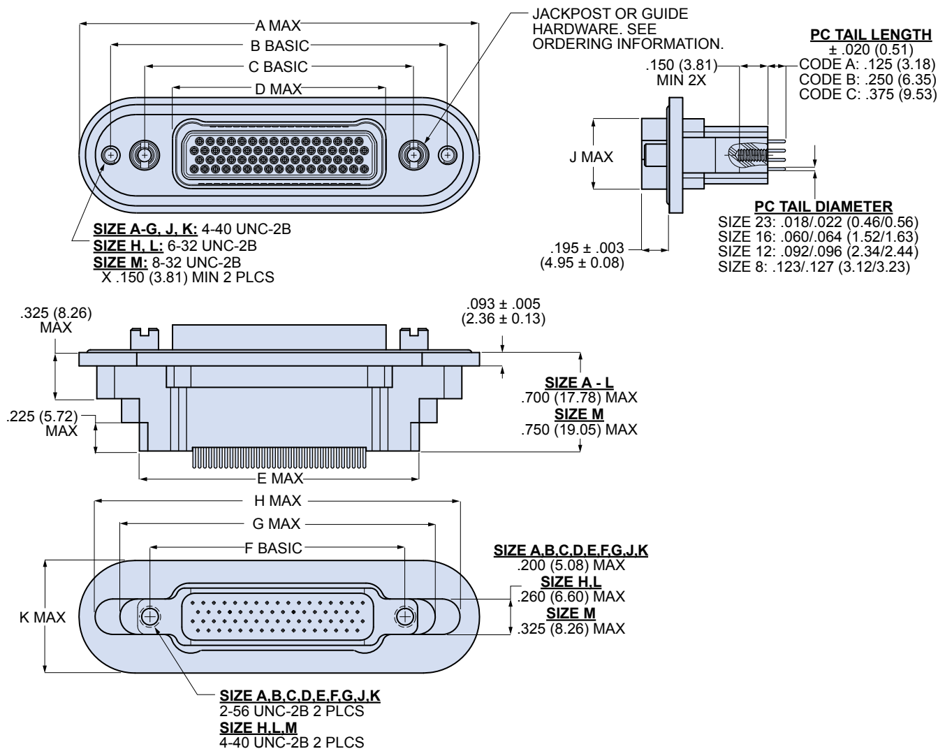
791-021P Dimensions
