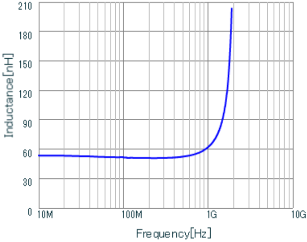
LQP03HQ51NH02 L.
