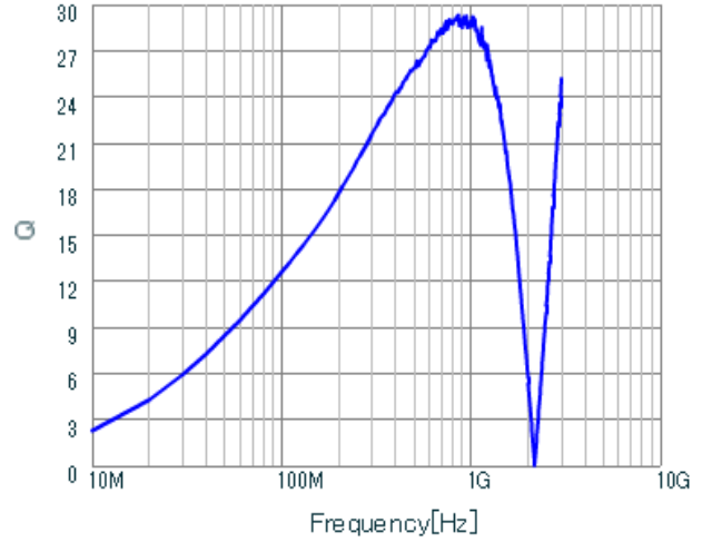
LQP03HQ51NH02 Q.
