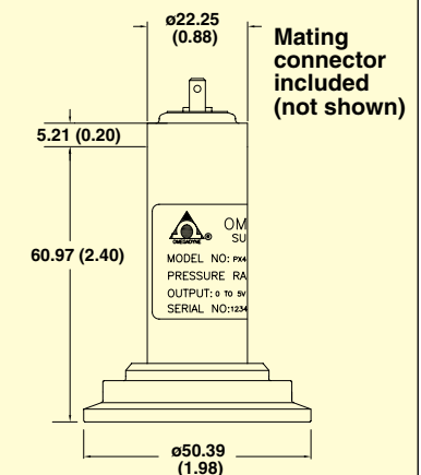
PX419S15 1½" flange
