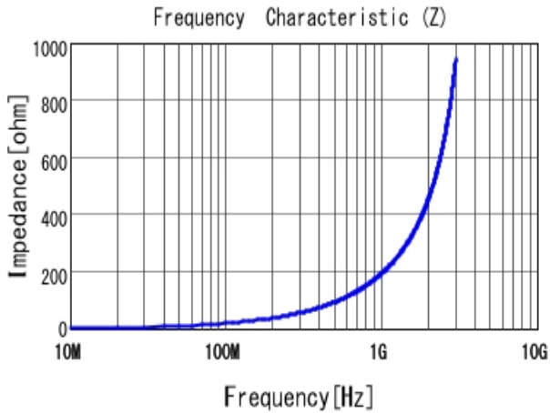
■ LQW15AN30NG00 |Z|
