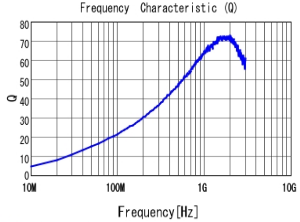
■ LQW15AN30NG00 Q
