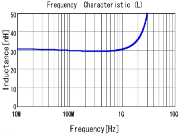
■ LQW15AN30NG00 L
