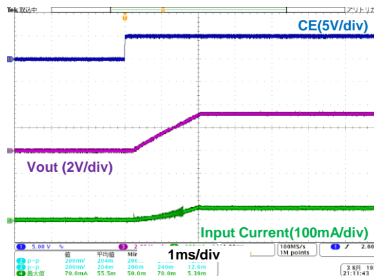
(5-4) Vin = 24V, Iout = 300mA
