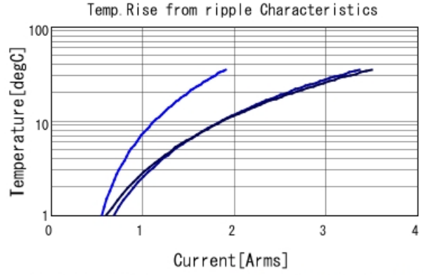
GCJ31CR71H105KA12 Temp. rise ■ 100kHz ■ 500kHz ■ 1MHz
