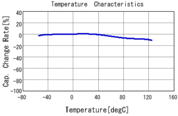
■ GCJ31CR71H105KA12 C-Temp. capchange, DCO. 0V, AC1. 0Vrm
