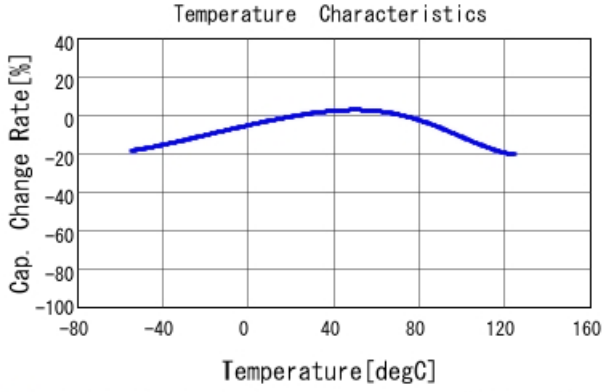
■ GRM31CC71C226ME11 C-Temp. capchange, DCO. 0V, ACO. 35Vr
