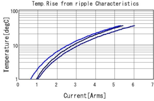
GRM31CC71C226ME11 Temp. rise ■ 80kHz ■ 400kHz ■ 800kHz
