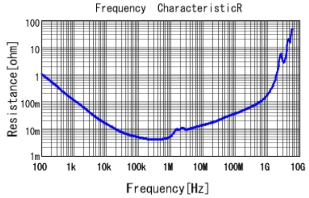
■ GCJ32ER70J476KE01 R DC0V, 25degC
