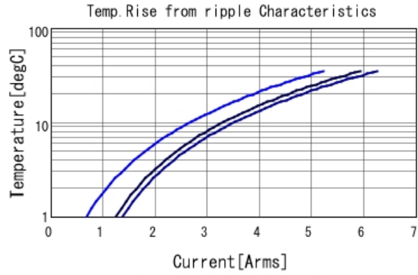
GCJ32ER70J476KE01 Temp. rise ■ 60kHz ■ 300kHz ■ 600kHz
