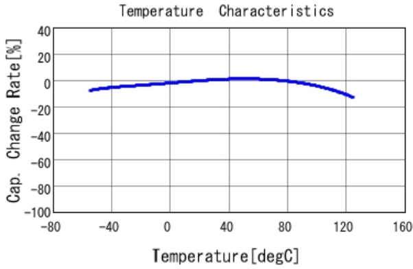
■ GCJ32ER70J476KE01 C-Temp. capchange, DCO. 0V, ACO. 5Vrm
