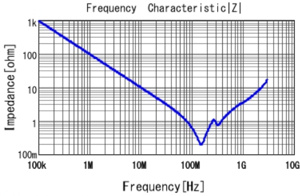
■ GA343QR7GD182KW01 |Z| DCOV, 25degC
