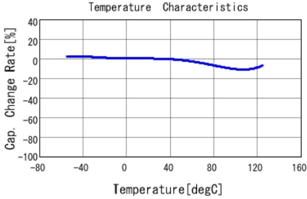
■ GA343QR7GD182KW01 C-Temp. capchange, DCOV, AC1Vrms
