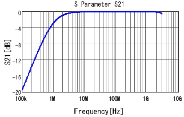
■ GA343QR7GD182KW01 S21 DCOV, 25degC
