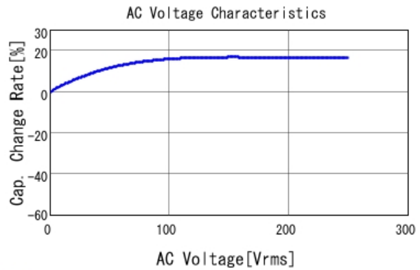
■ GA343QR7GD182KW01 C-AC Voltage capchange, DCOV, 25.0d
