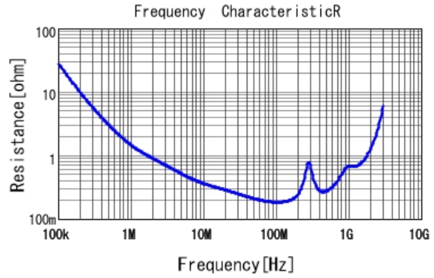
■ GA343QR7GD182KW01 R DCOV, 25degC
