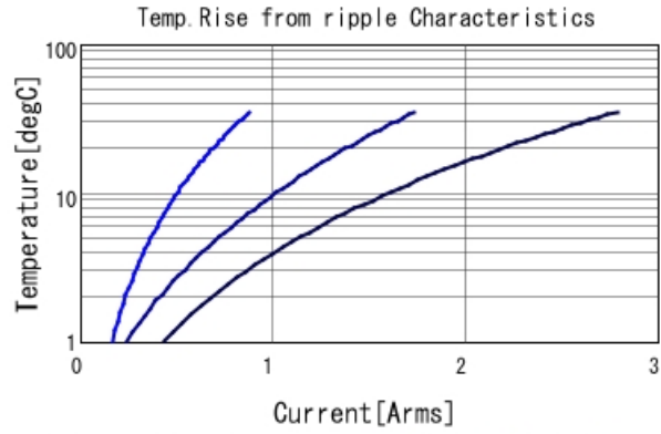
GC332DD72W104KX01 Temp. rise ■ 30kHz ■ 100kHz ■ 300kHz
