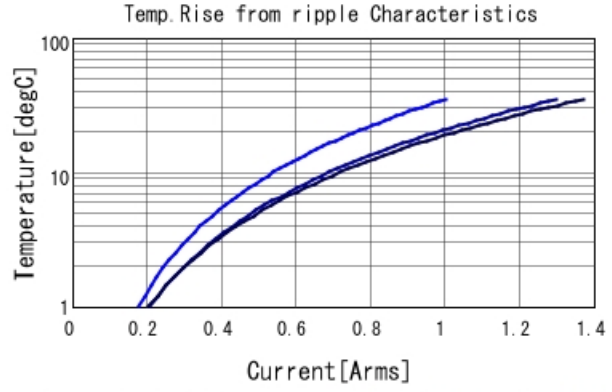
GCJ188R91H104KA01 Temp. rise ■ 400kHz ■ 800kHz ■ 1MHz
