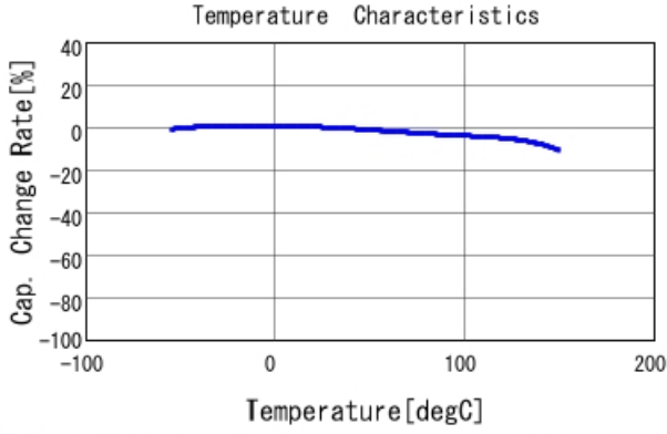
■ GCJ188R91H104KA01 C-Temp. capchange, DCO. 0V, AC1. 0Vrm
