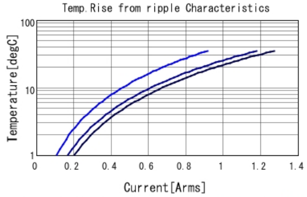
GCJ188R91H124KA01 Temp. rise ■ 400kHz ■ 800kHz ■ 1MHz
