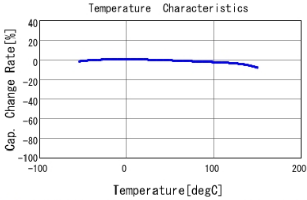
■ GCJ188R91H124KA01 C-Temp. capchange, DCO. 0V, AC1. 0Vrm
