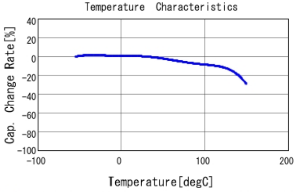
■ GCJ21BL81E684KA01 C-Temp. capchange, DCO. 0V, AC1. 0Vrm
