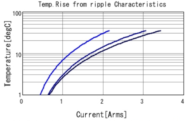
GCJ21BL81E684KA01 Temp. rise ■ 200kHz ■ 500kHz ■ 1MHz
