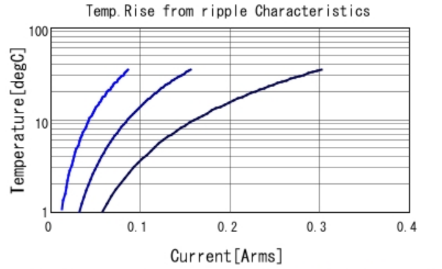
GCJ31BR72J472KXJ1 Temp. rise ■ 30kHz ■ 100kHz ■ 300kHz
