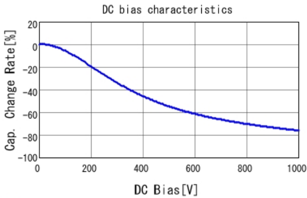
■ GCJ31BR73A152KXJ1 C-DC bias capchange, 25.0degC, AC1V
