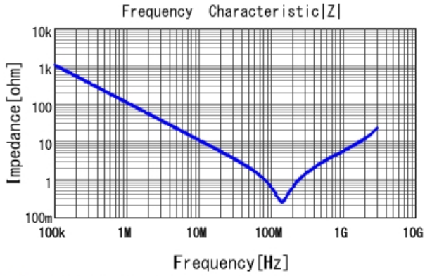
■ GCJ31BR73A152KXJ1 |Z| DC0V, 25degC
