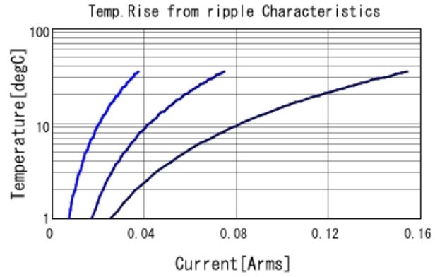
GCJ31BR73A152KXJ1 Temp. rise ■ 30kHz ■ 100kHz ■ 300kHz
