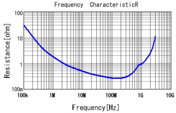
■ GCJ31BR73A152KXJ1 R DC0V, 25degC
