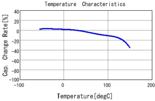
■ GCJ31CL81C335KA01 C-Temp. capchange, DCO. 0V, AC1. 0Vrm
