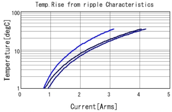
GCJ31CL81C335KA01 Temp. rise ■ 100kHz ■ 500kHz ■ 1MHz
