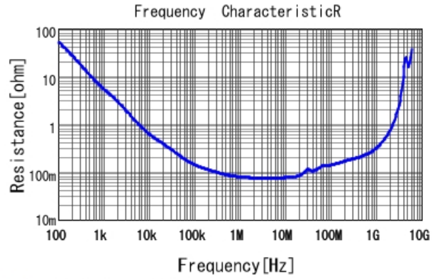
■ GCJ31MR72A154KA01 R DCOV, 25degC
