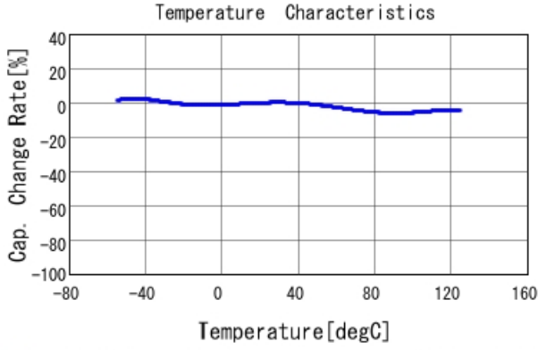
■ GCJ31MR72A154KA01 C-Temp. capchange, DCO. 0V, AC1. 0Vrm
