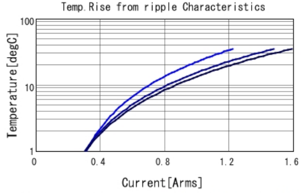
GCJ31MR72A154KA01 Temp. rise ■ 400kHz ■ 800kHz ■ 1MHz
