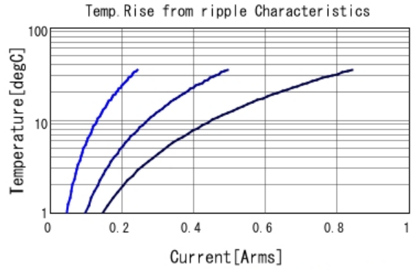
GCJ43DR73A333KXJ1 Temp. rise ■ 30kHz ■ 100kHz ■ 300kHz
