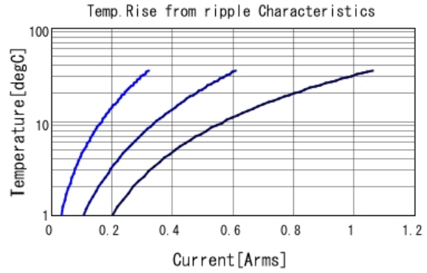
GCJ43DR73A473KXJ1 Temp. rise ■ 30kHz ■ 100kHz ■ 300kHz
