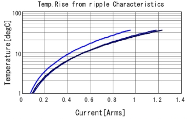
GCM155R71C154KE02 Temp. rise ■ 400kHz ■ 800kHz ■ 1MHz
