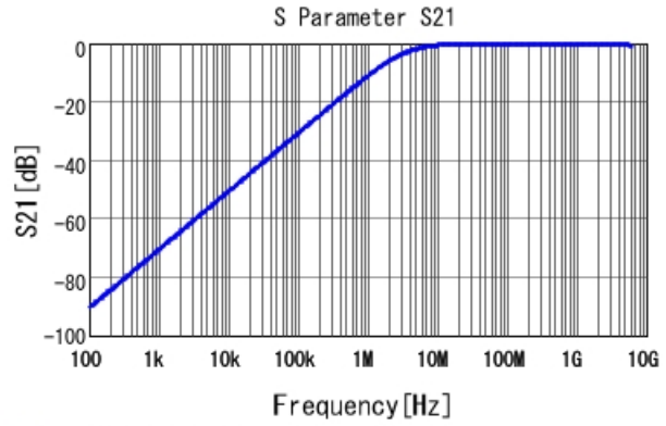
■ GCM155R71H471KA37 S21 DCOV, 25degC
