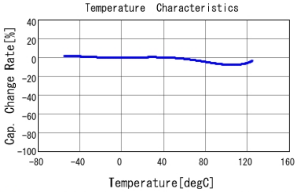
■ GCM155R71H471KA37 C-Temp. capchange, DCO. 0V, AC1. 0Vrm
