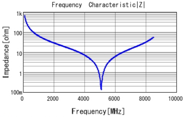
■ GQM2195G2E2R4WB12 |Z| DC0V, 25degC
