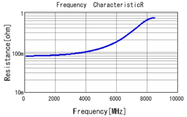
■ GQM2195G2E2R4WB12 R DC0V, 25degC
