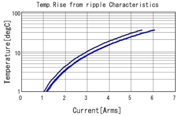
GRJ32EC71E226KE11 Temp. rise ■ 80kHz ■ 400kHz ■ 800kHz
