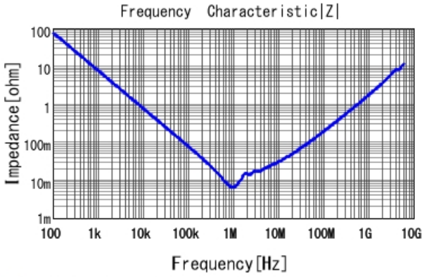
■ GRJ32EC71E226KE11 |Z| DC0V, 25degC
