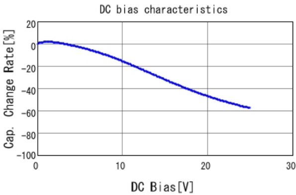
■ GRJ32EC71E226KE11 C-DC bias capchange, 25.0degC, AC0.
