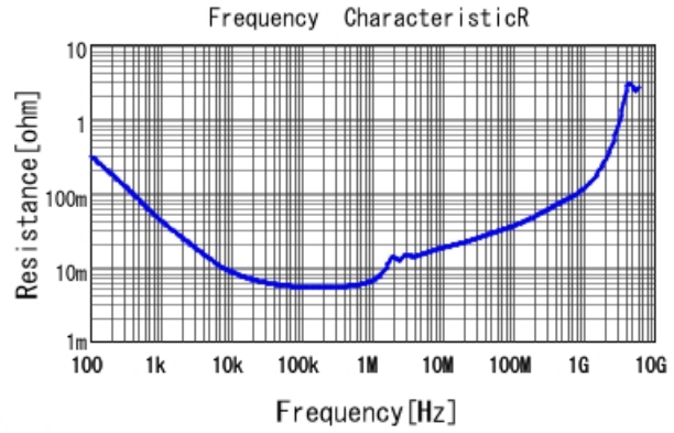
■ GRJ32EC71E226KE11 R DC0V, 25degC
