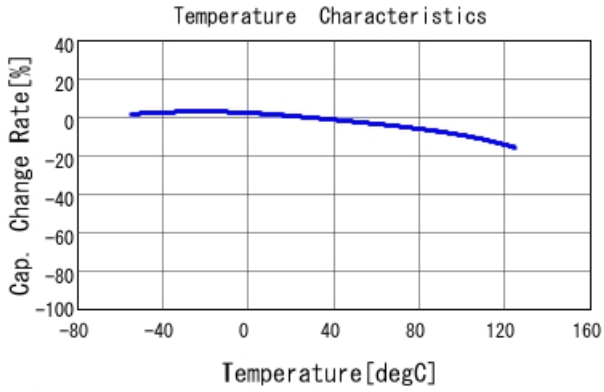
■ GRJ32EC71E226KE11 C-Temp. capchange, DCO. 0V, ACO. 5Vrm
