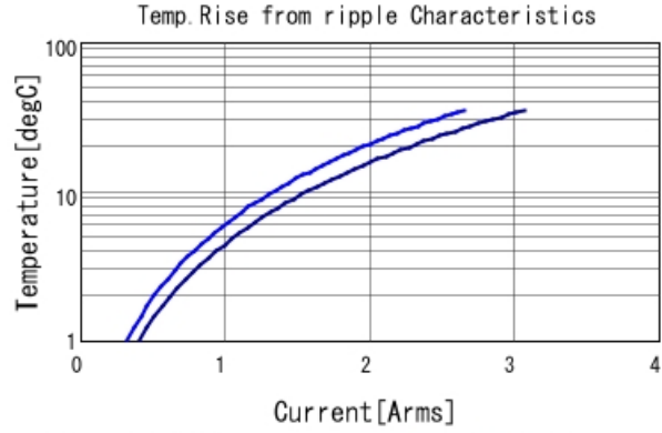
GRM155C81C105KE11 Temp. rise ■ 500kHz ■ 1MHz
